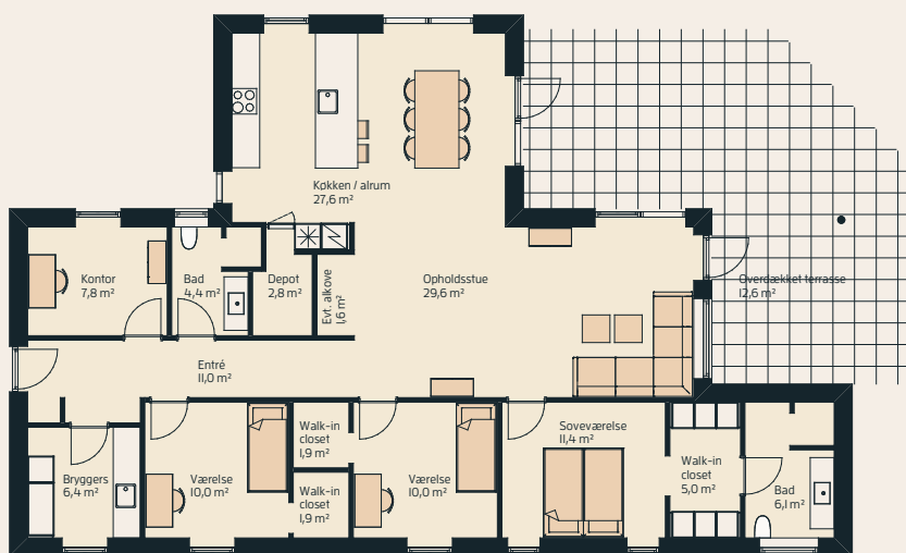
Vinkelhus 168 m 2
